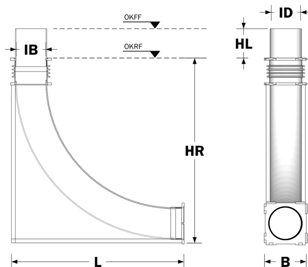
Technische Zeichnung (Gebäudeeinführung)
