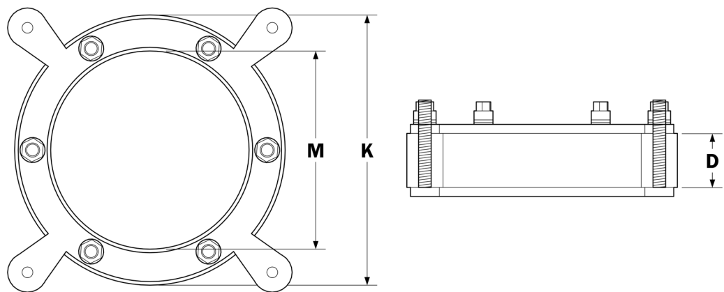
Technische Zeichnung
