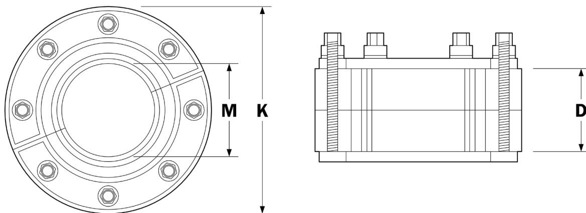
Technische Zeichnung
